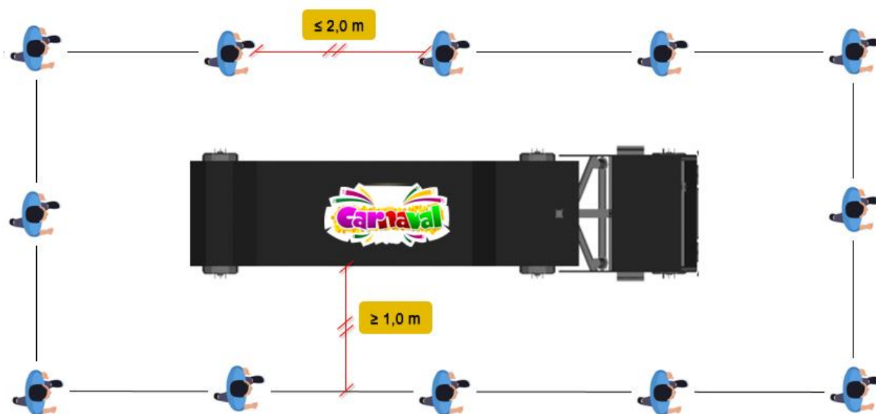
Figura A.5 – Veículo do tipo pranchão/"trem elétrico" 1
